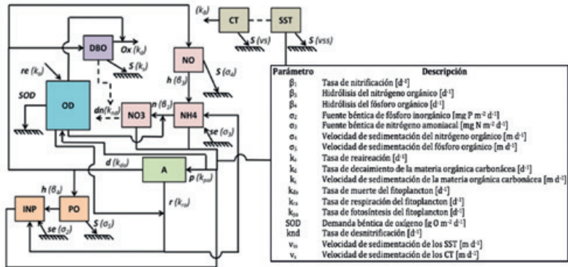
Figura 7. Ejemplo de esquema conceptual de procesos de calidad del agua
