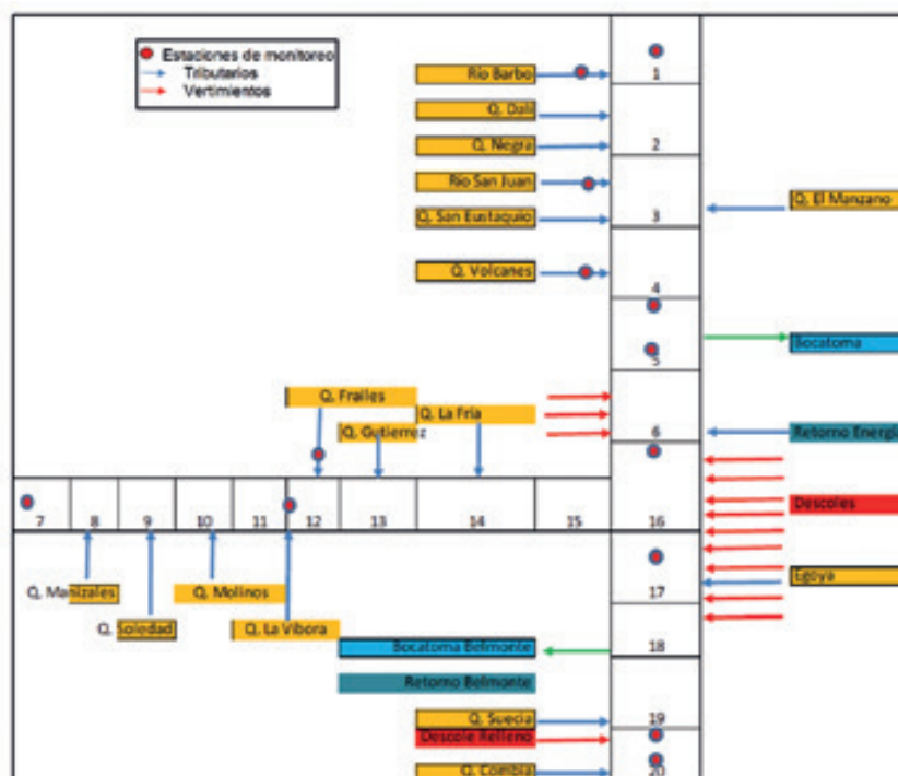
Figura 6. Ejemplo de esquematización del sistema, incluyendo entradas, salidas, puntos de monitoreo y segmentación de cuerpos de agua
