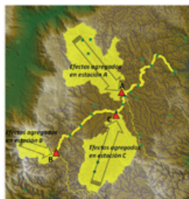
Figura 14. Esquema de modelación de calidad del agua a escala regional
