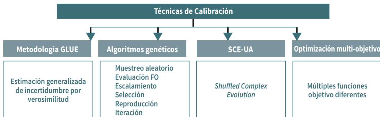
Figura 12. Técnicas de calibración de uso común para modelos de calidad del agua
